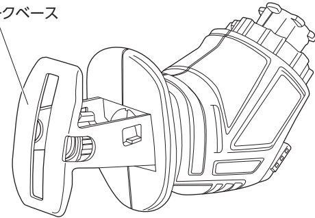
電気のこぎりユニット×1
