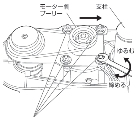
ベルトテンション調節ナット (4ヶ所あります)
